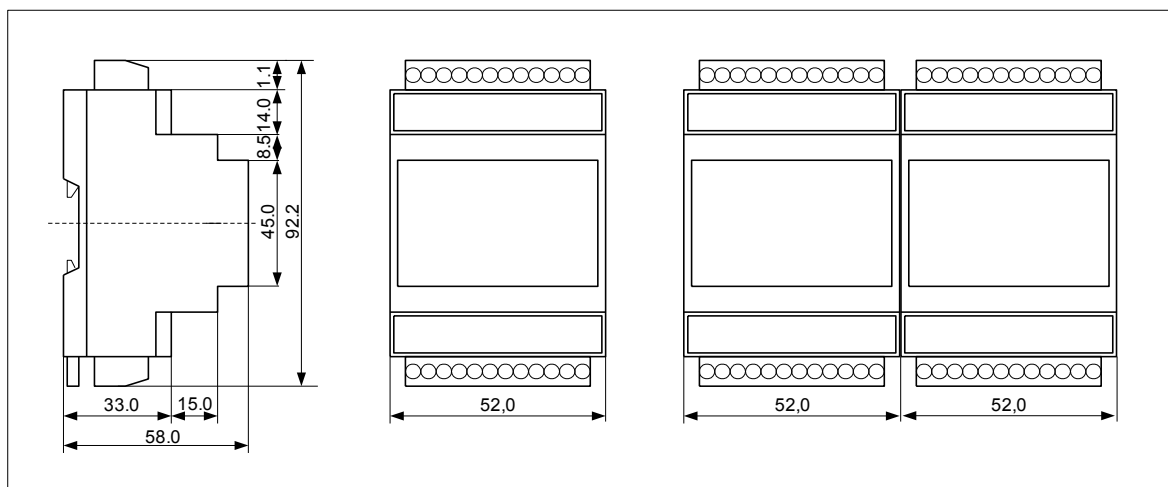
Rys. 2.5.1. Wymiary modułu CM-180
