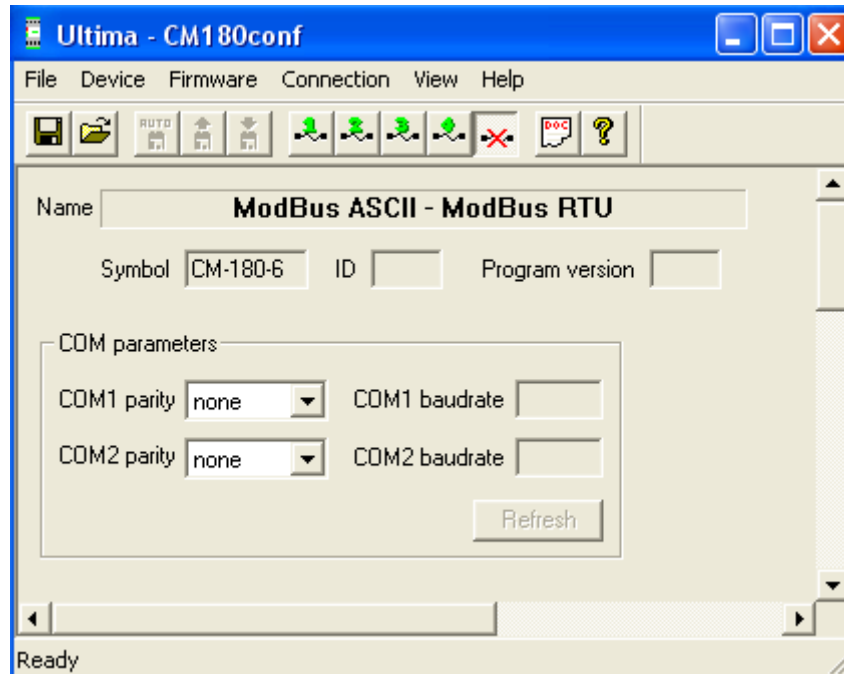
Rys 4.3.3.1. Parametry konfiguracyjne urządzenia CM-180-6
