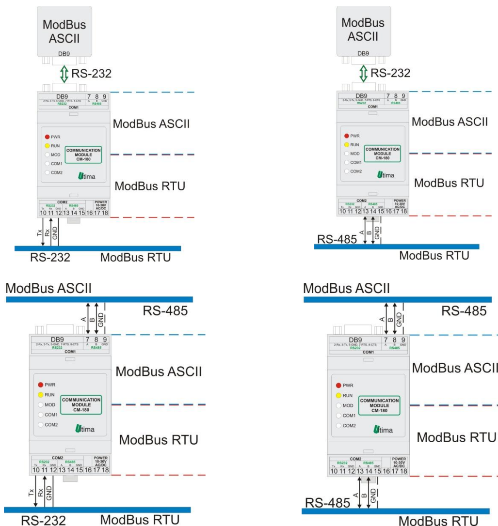
Rys.4.3.2.1. Sposoby podłączenia CM-180-6
