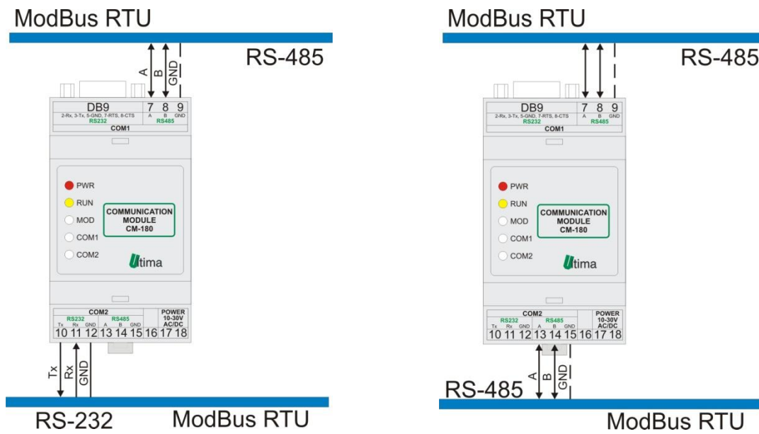
Rys.4.3.2.1. Sposoby podłączenia CM-180-3
