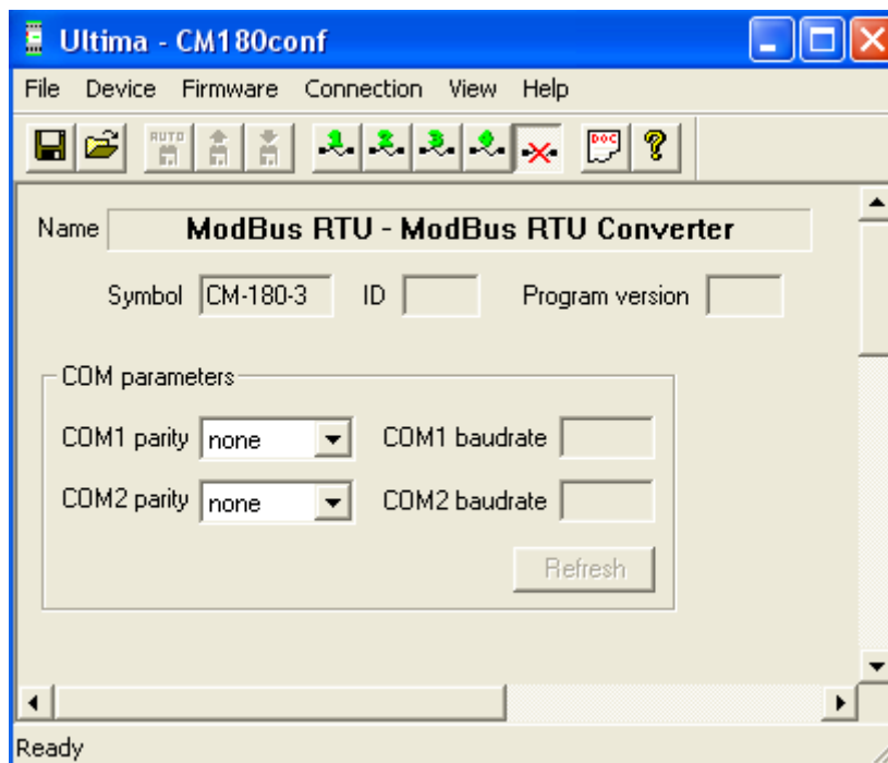
Rys 4.3.3.1. Parametry konfiguracyjne urządzenia CM-180-3
