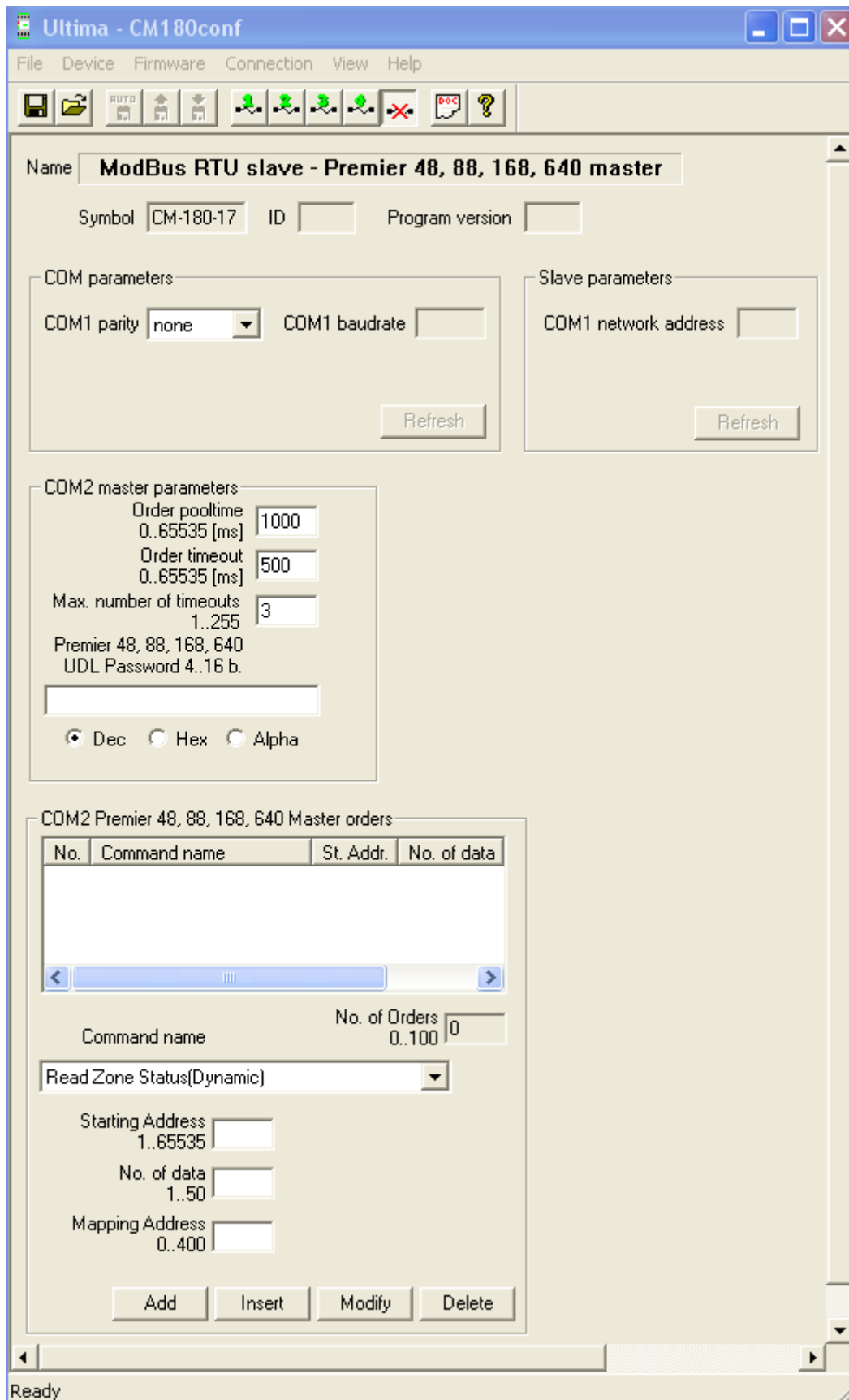
Rys 4.3.3.1. Parametry konfiguracyjne urządzenia CM-180-17
