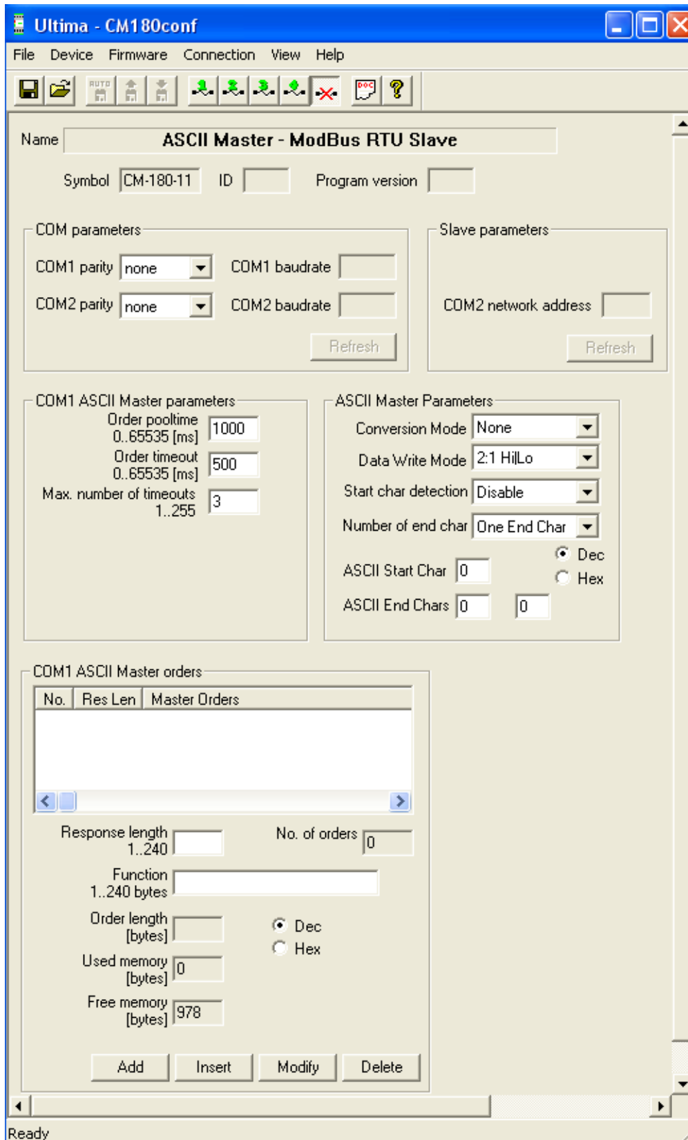
Rys 4.3.3.1. Parametry konfiguracyjne urządzenia CM-180-11
