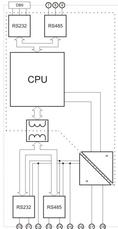
Rys2.2.1. Schemat blokowy modułu CM-180
