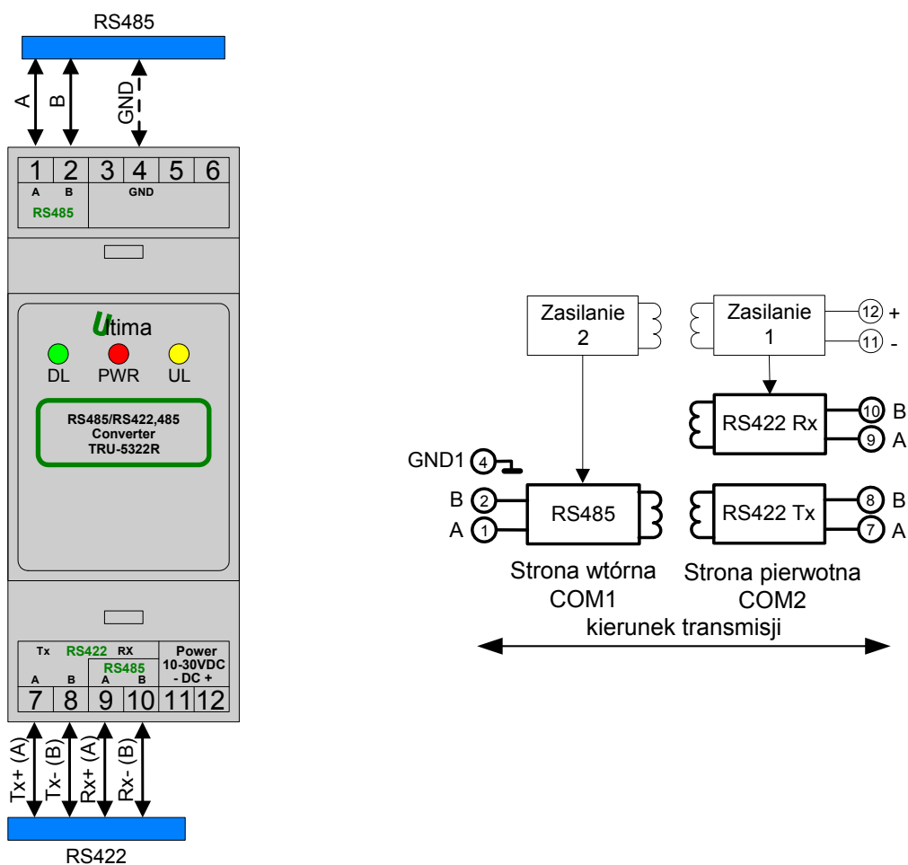
Rys. 3.1 Konwerter TRU-5322R w konfiguracji RS485 na RS422 oraz RS422 na RS485
