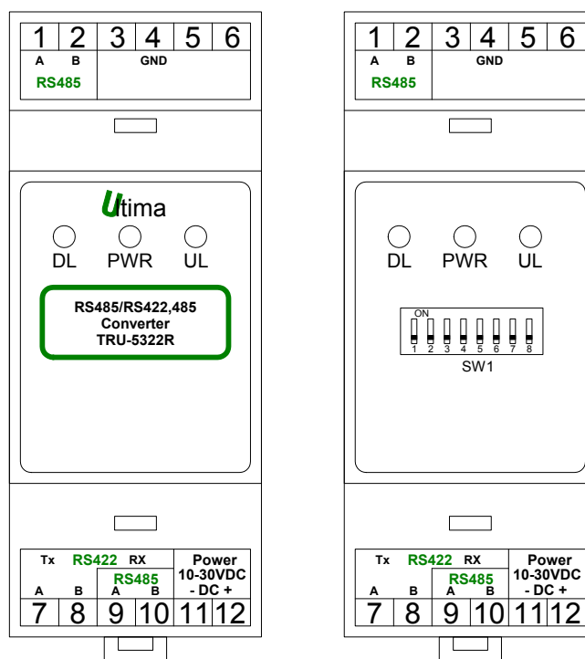
Rys. 2.2 Widok złącz konwertera TRU-5322R od frontu
