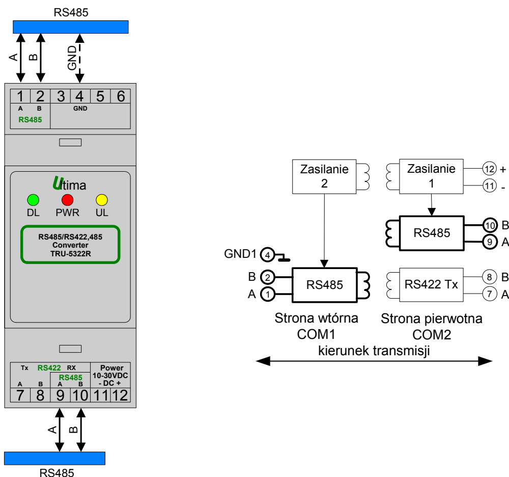
Rys. 3.2 Konwerter TRU-5322R w konfiguracji wzmacniacza, separatora RS485 na RS485
