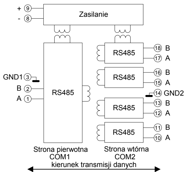
Rys. 2.1 Schemat blokowy modułu HRU-5330R
