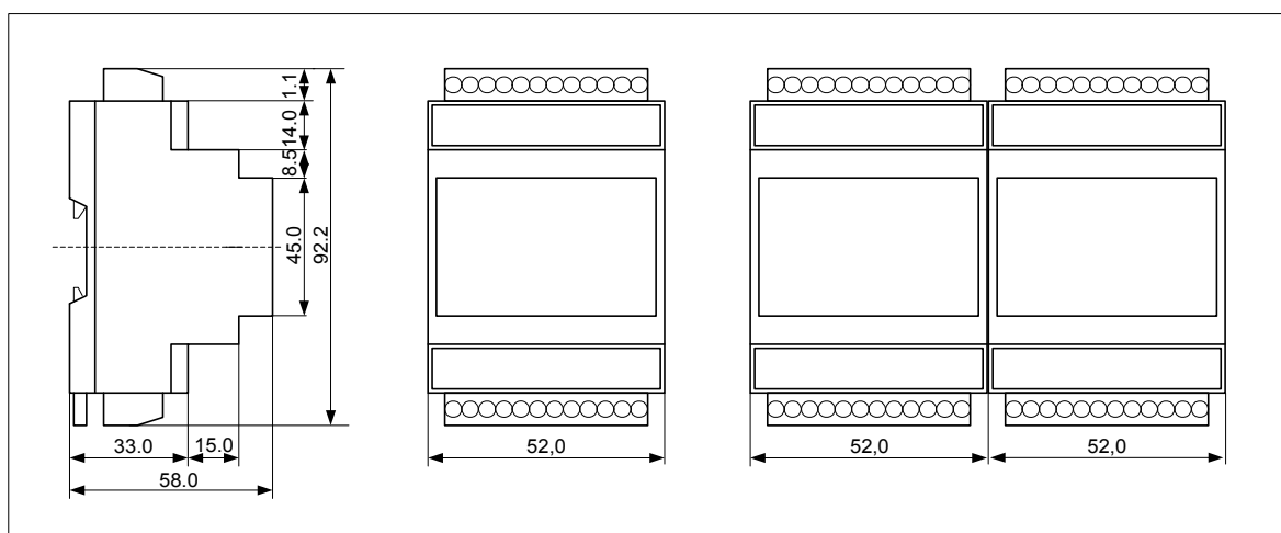
Rys. 2.4 Wymiary modułu HRU-5330R
