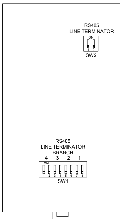
Rys. 2.3 Widok złączy modułu HRU-5330R od tyłu
