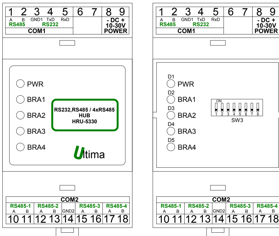
Rys. 2.2 Widok złącz modułu HRU-5330R od frontu
