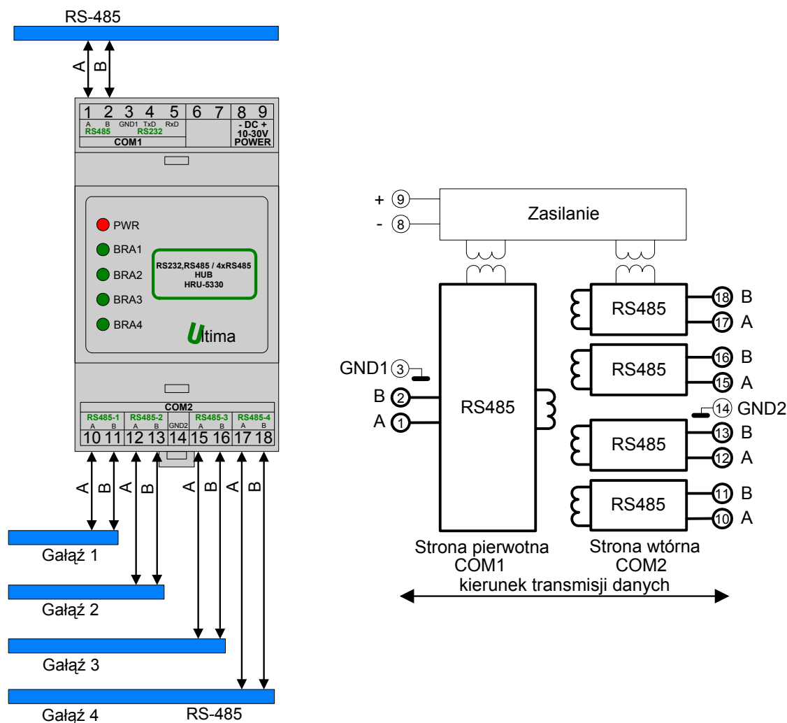
Rys. 3.1 Sposób połączenia modułu HRU-5330R jako HUB-separator RS485 na 4x RS485
