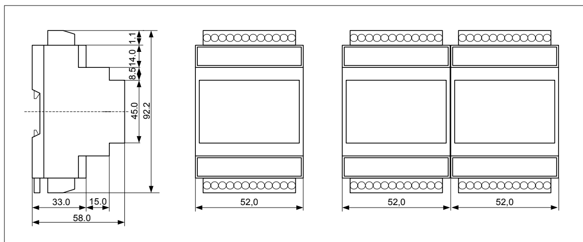
Rys. 2.4 Wymiary modułu HRU-5330
