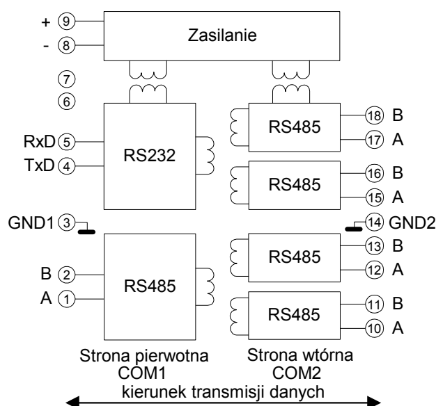
Rys. 2.1 Schemat blokowy modułu HRU-5330
