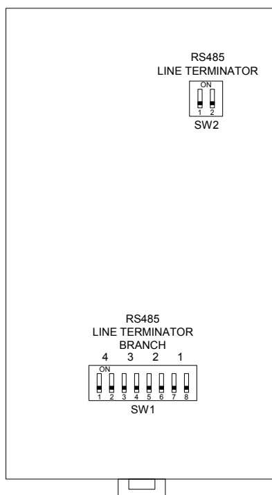
Rys. 2.3 Widok złącz modułu HRU-5330 od tyłu
