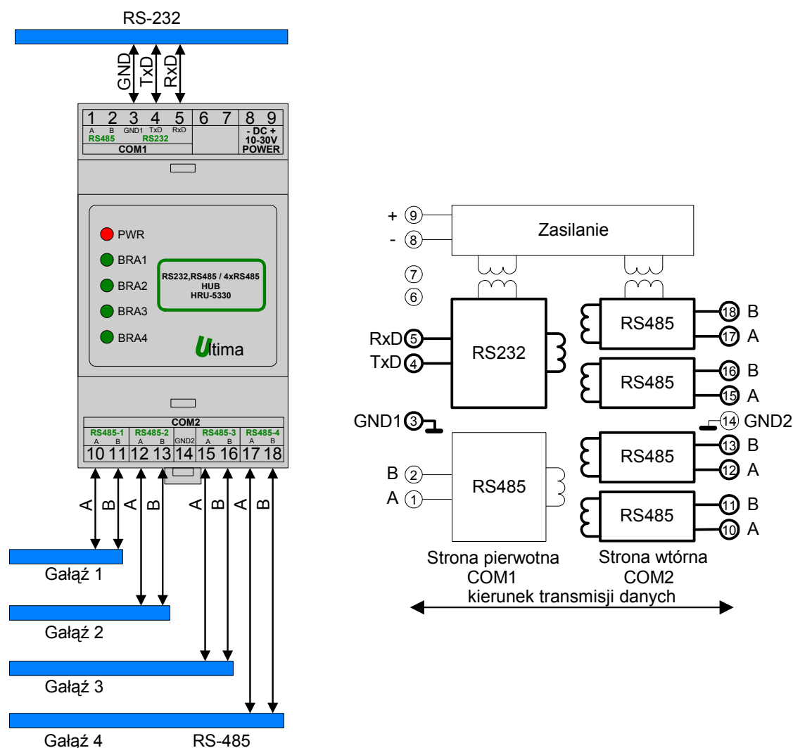
Rys. 3.2 Sposób połączenia modułu HRU-5330 jako HUB-konwerter RS232 na 4x RS485
