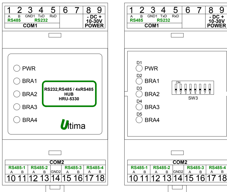
Rys. 2.2 Widok złącz modułu HRU-5330 od frontu
