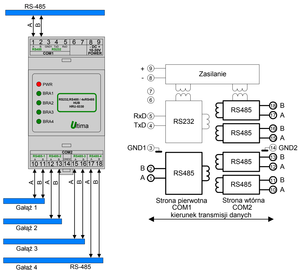
Rys. 3.1 Sposób połączenia modułu HRU-5330 jako HUB-separator RS485 na 4x RS485
