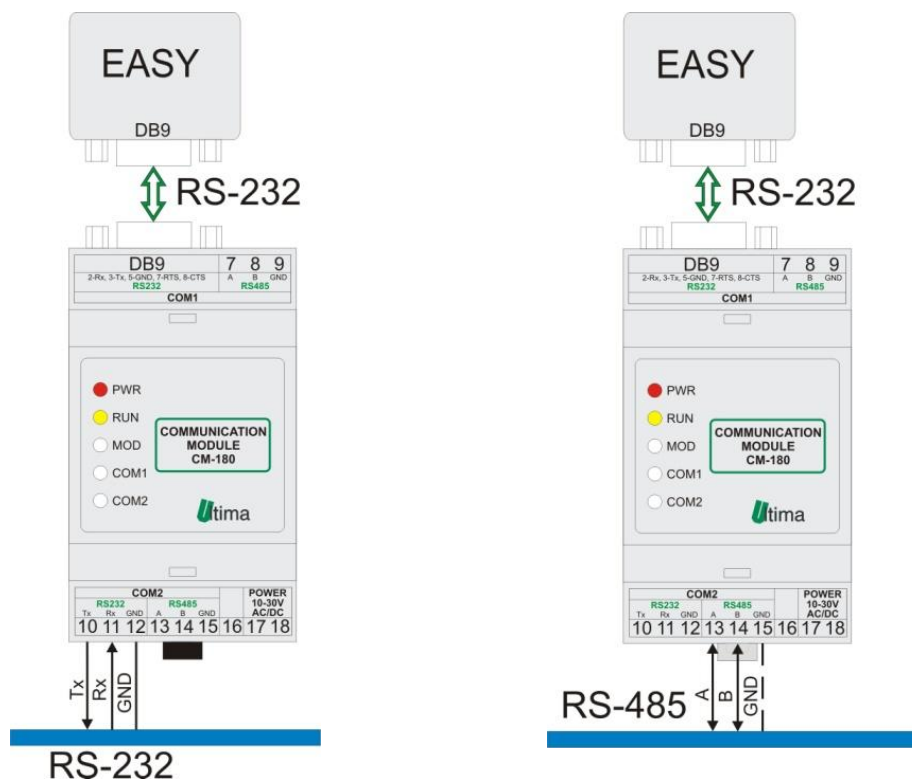
Rys.4.3.2.1. Sposoby podłączenia CM-180-9
