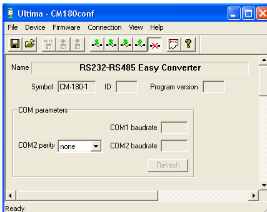
Rys 4.3.3.1. Parametry konfiguracyjne urządzenia CM-180-1
