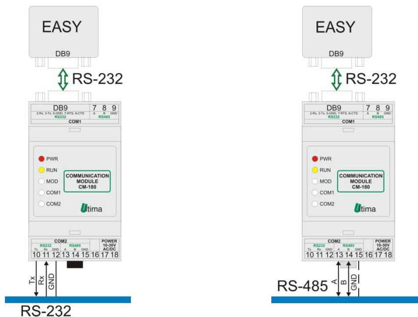
Rys.4.3.2.1. Sposoby podłączenia CM-180-1
