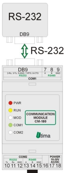
Rys. 4.1.2. Podłączenie modułu w trybie programowania
